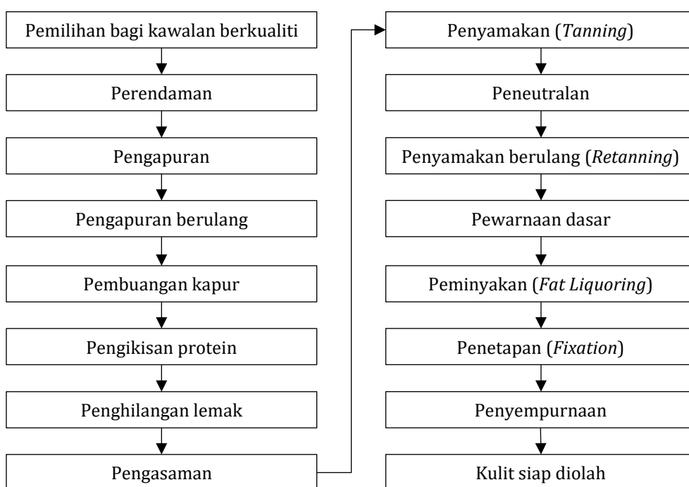
Rajah 1 Carta proses pengolohan kulit melalui proses samak (MS 2200-2 (2012))
